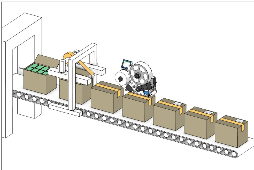
Tabakproduktionslinie mit integriertem Videojet® 9550-Etikettendruckspendensystem mit DirectApply™-Technologie.
