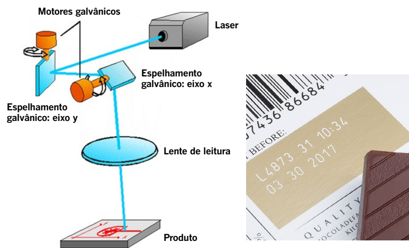
Diagrama da tecnologia de laser CO 2
